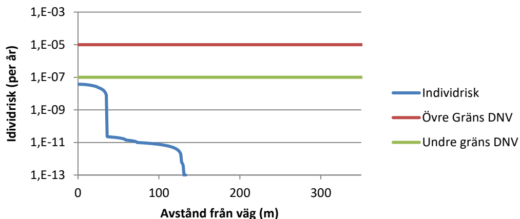
Figur 15. Individrisk längs med Mensättravägen med varierad indata.
