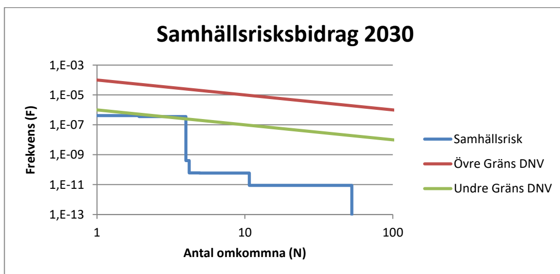
Figur 14. Samhällsrisk för nuläge med ny bebyggelse år 2030.
