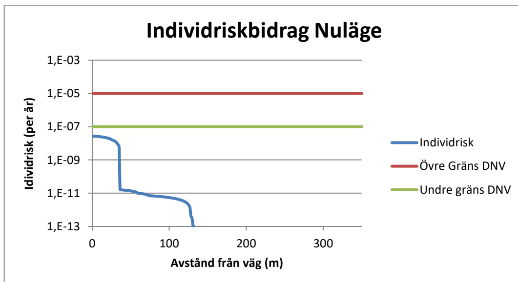
Figur 11. Individrisk längs med Mensättravägen för nuläge med trafik från ny bebyggelse.
