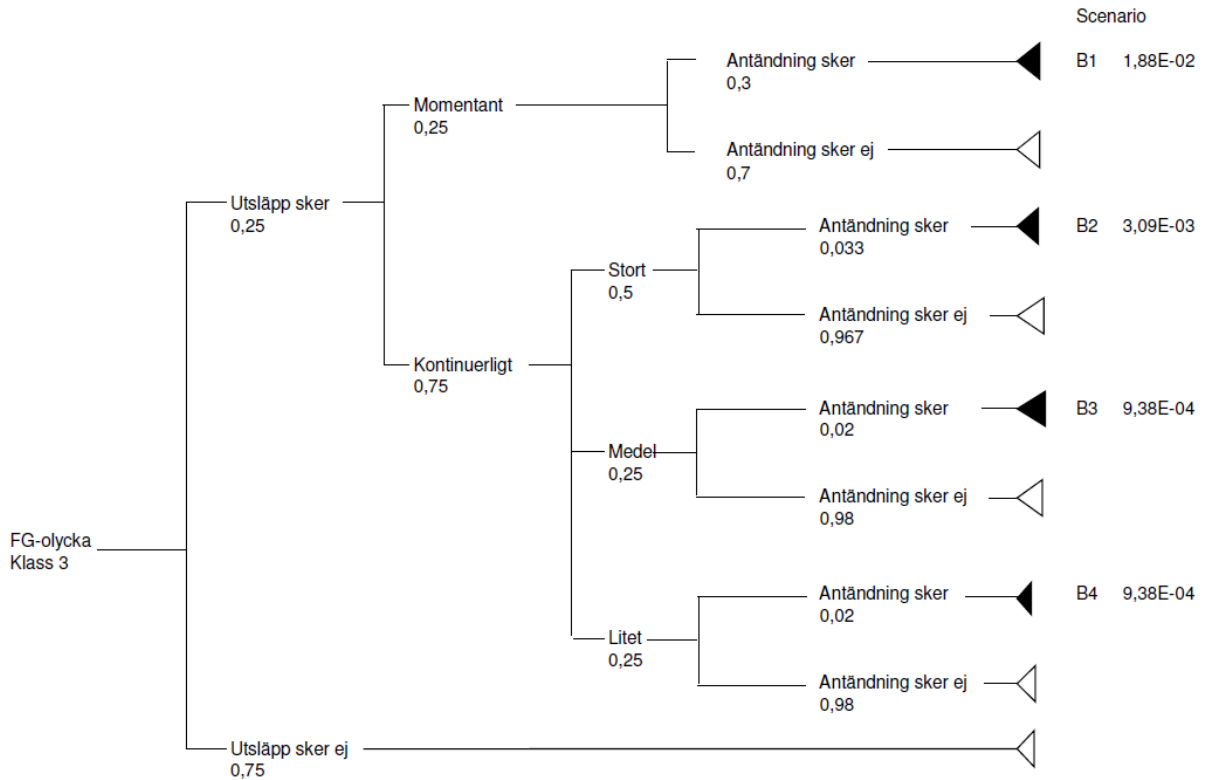
Figur A.2.2. Händelseträd över farligt godsolycka med klass 3.
